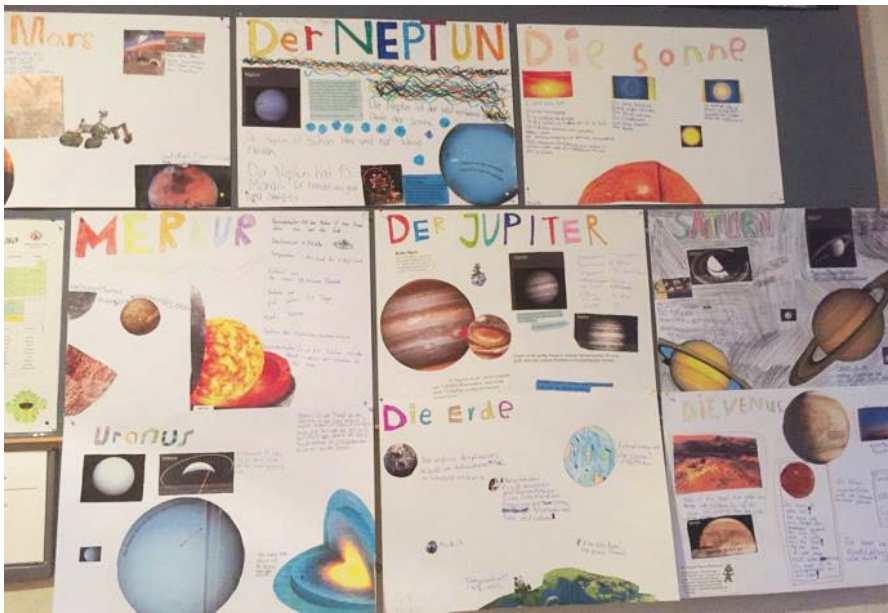
Die bunten Plakate der Planeten unseres Sonnensystems.
